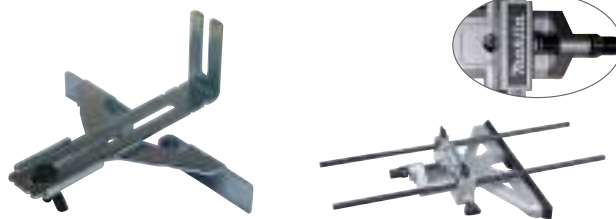
Guia paralela com ajuste milimétrico
